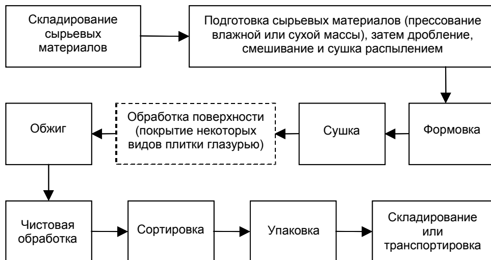
Рисунок А.1. Типичный процесс производства керамической плитки
