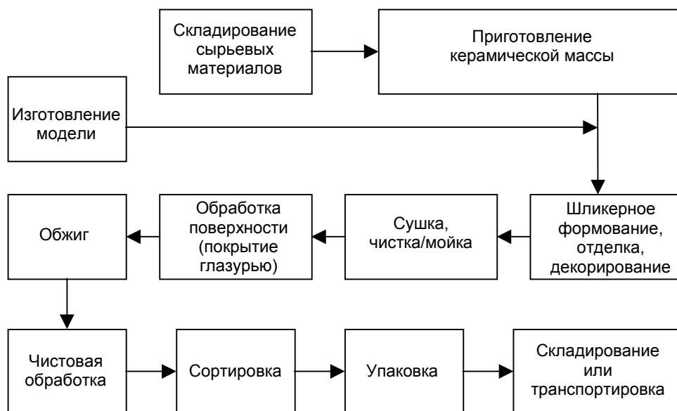
Рисунок А.2. Типичный процесс производства санитарно-технических изделий
