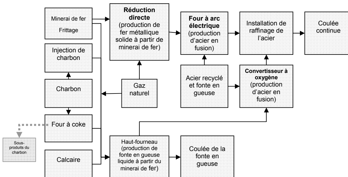
Figure A.1 Processus de production des aciéries intégrées
