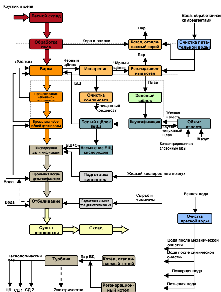
Рисунок 1. Сульфатный метод производства целлюлозы
